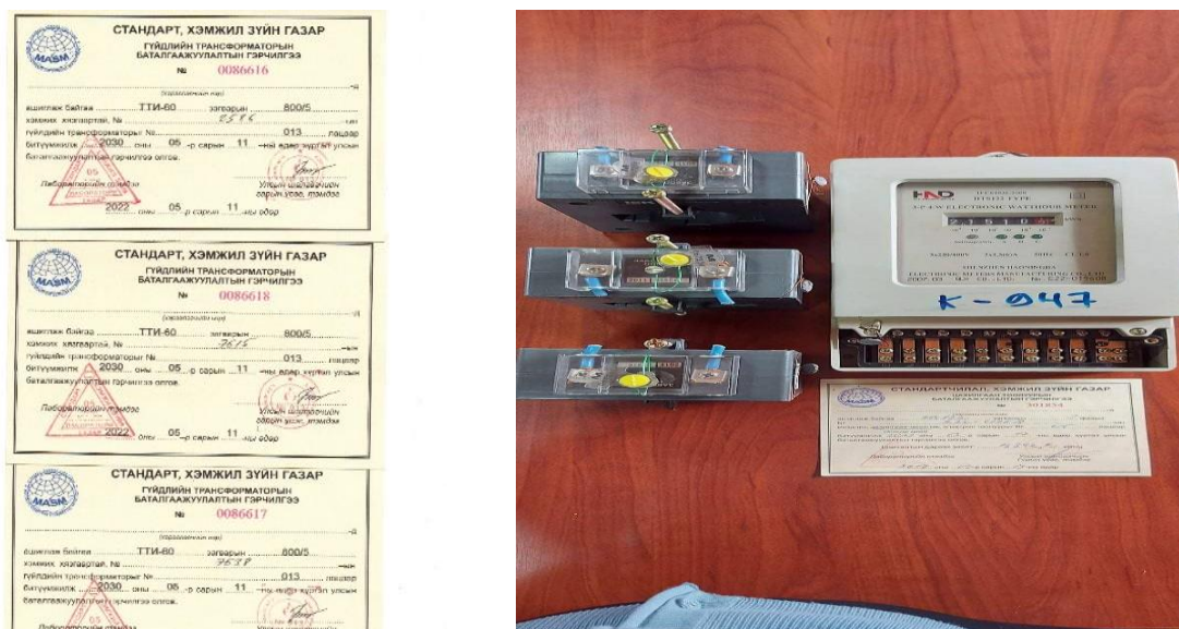
Зураг 5. Цахилгааны тоолуур, гүйдлийн трансформатор
